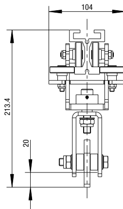
フォーホールドヘビーデューティーキャリア260=HD260 / Fourfold Heavy Duty Carrier 260 = HD260
