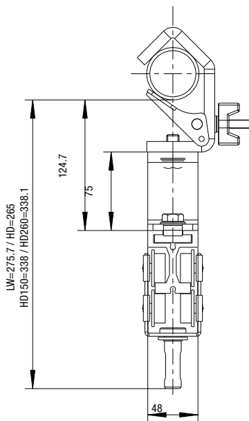
ダブルヘビーデューティーキャリア150=HD150 / Double Heavy Duty Carrier 150 = HD150
