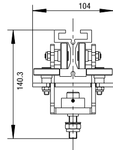
HDキャリア=HD / HD Carrier = HD
