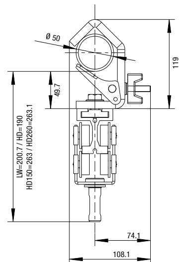
直接トラック取付 / Direct track mounting
