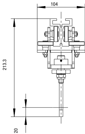
ダブルヘビーデューティーキャリア150=HD150 / Double Heavy Duty Carrier 150 = HD150
