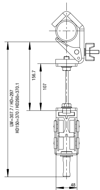
ダブルトップコードオペレーション / Double Top Cord Operation
